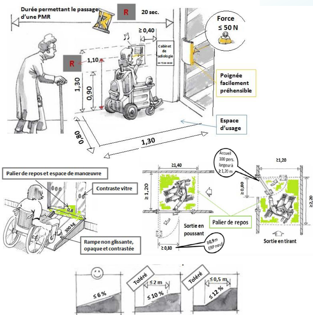
Valeurs de pente pour rampe d'accès
